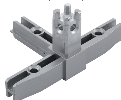
4 x łącznik narożny 4sh
