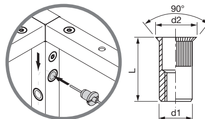
Nitonakrętka - linka/uchwyt
