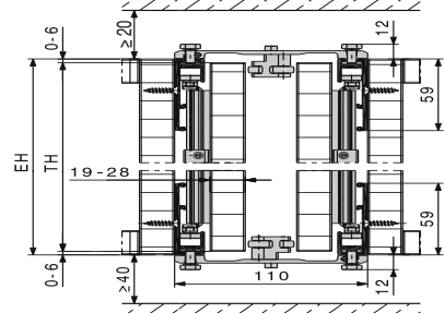
System: HAWA-Concepta 25/30 Połączenie: Profil Connector 110 mm
