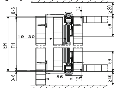
System: HAWA-Concepta 25/30 Połączenie: Profil Connector 55 mm
