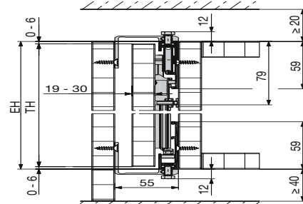
System: HAWA-Concepta 40/50 Połączenie: Profil Connector 55 mm
