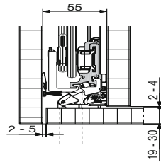
Connector 55 mm Maksymalna grubość drzwi: 30 mm
