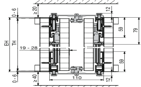
System: HAWA-Concepta 40/50 Połączenie: Profil Connector 110 mm
