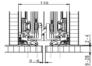
Connector 110 mm Maksymalna grubość drzwi: 28 mm
